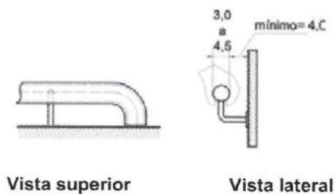
Figura 85 — Empunhadura de corrimão - Exemplo
