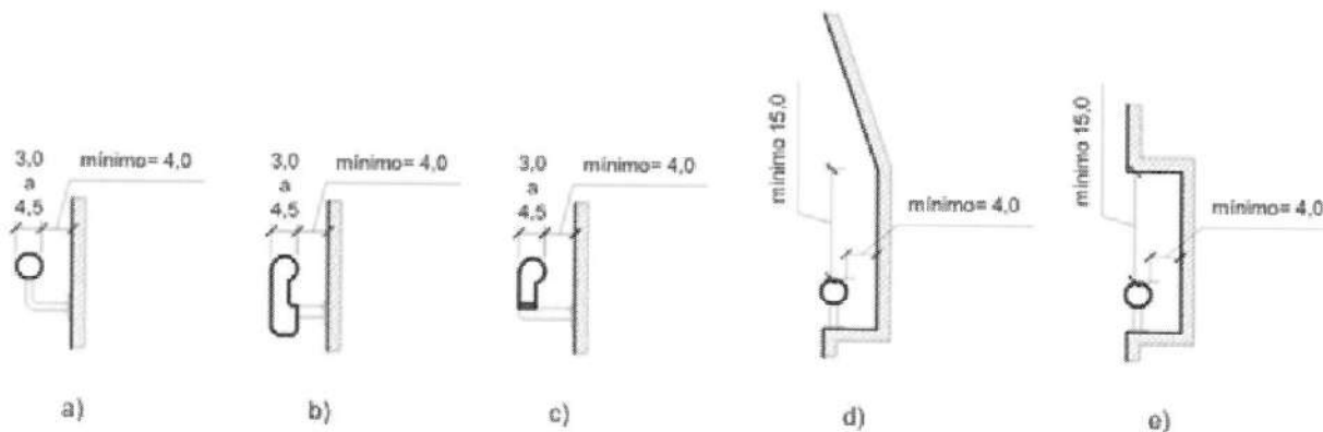
Figura 15 — Empunhadura
