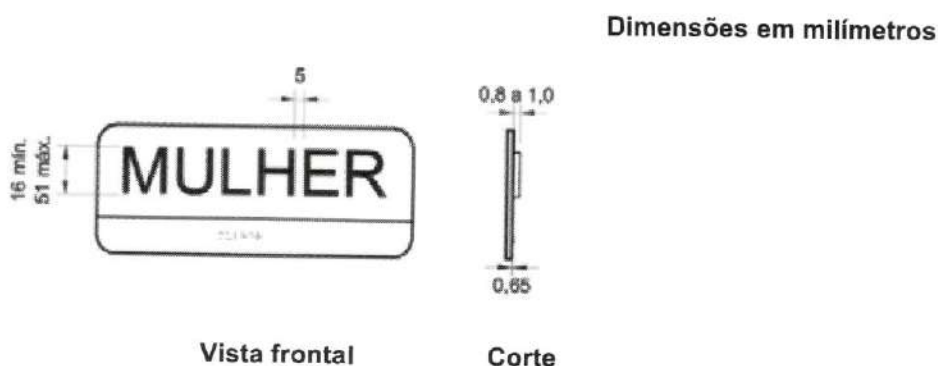
Figura 54 — Sinalização tátil – Exemplo
