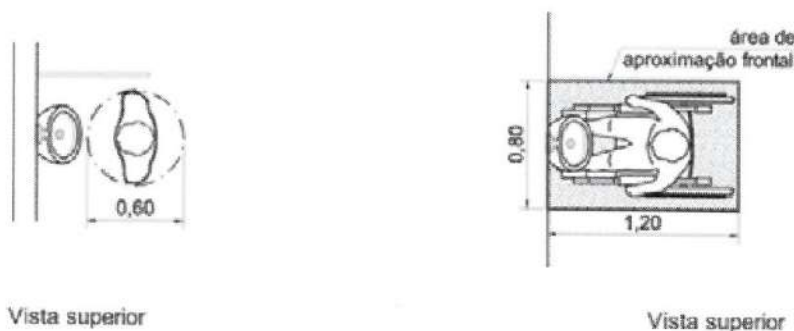
Figura 138 — Área de aproximação para P.M.R. Figura 139 — Área de aproximação para P.C.R.
