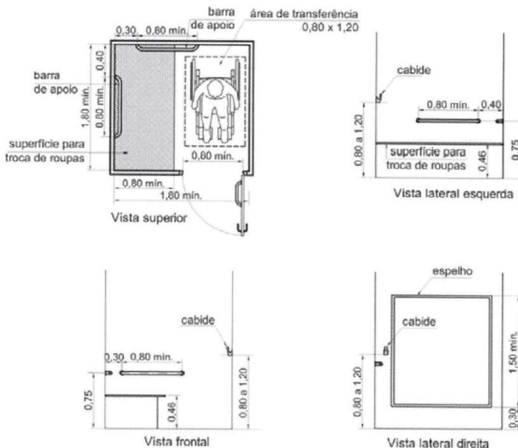
Figura 145 — Cabina para vestiário acessível — Exemplo
