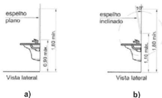
Figura 142 — Acessórios sanitários — Espelhos
