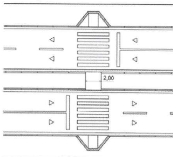
Figura 107 — Canteiro divisor de pistas - Exemplo 2
