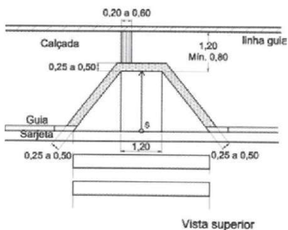
Figura 70 – Composição de sinalização tátil de alerta e direcional nos rebaixamentos das calçadas – Exemplo
