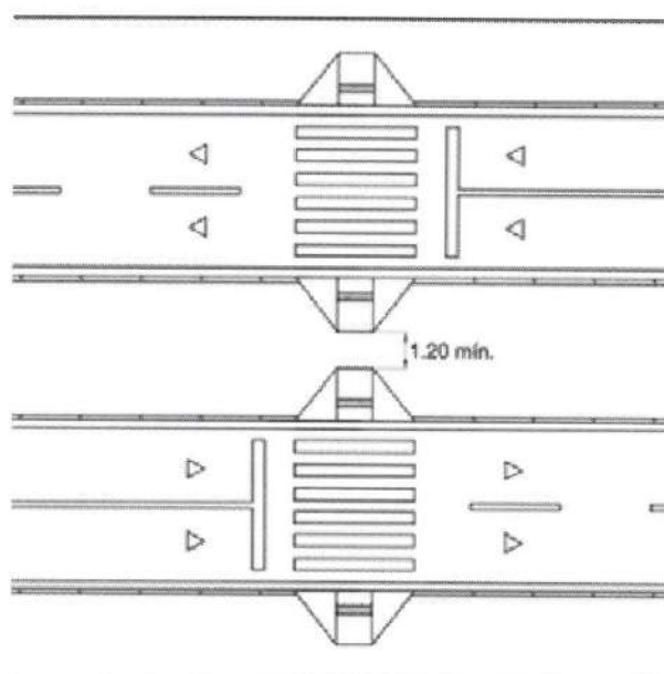
Figura 106 — Canteiro divisor de pistas - Exemplo 1
