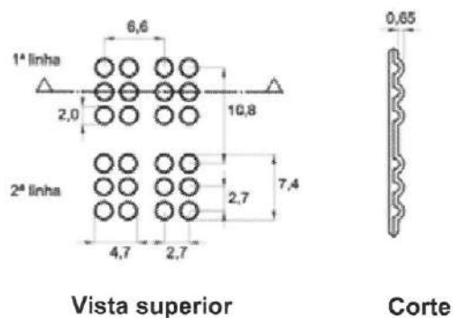
Figura 53 — Cela Braille
